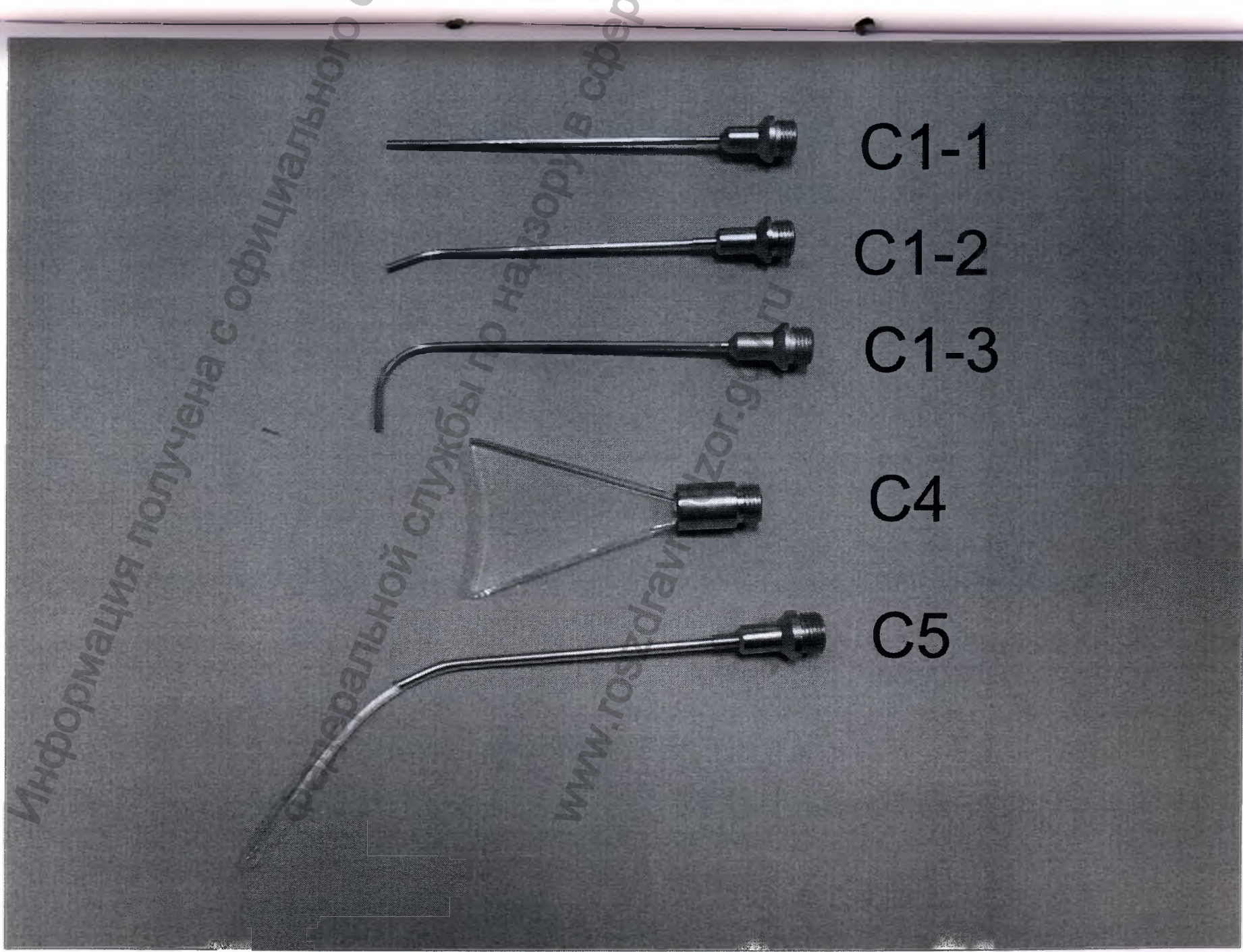
Насадки для стоматологии - C1-1, C1-2, C1-3, C4, C5
