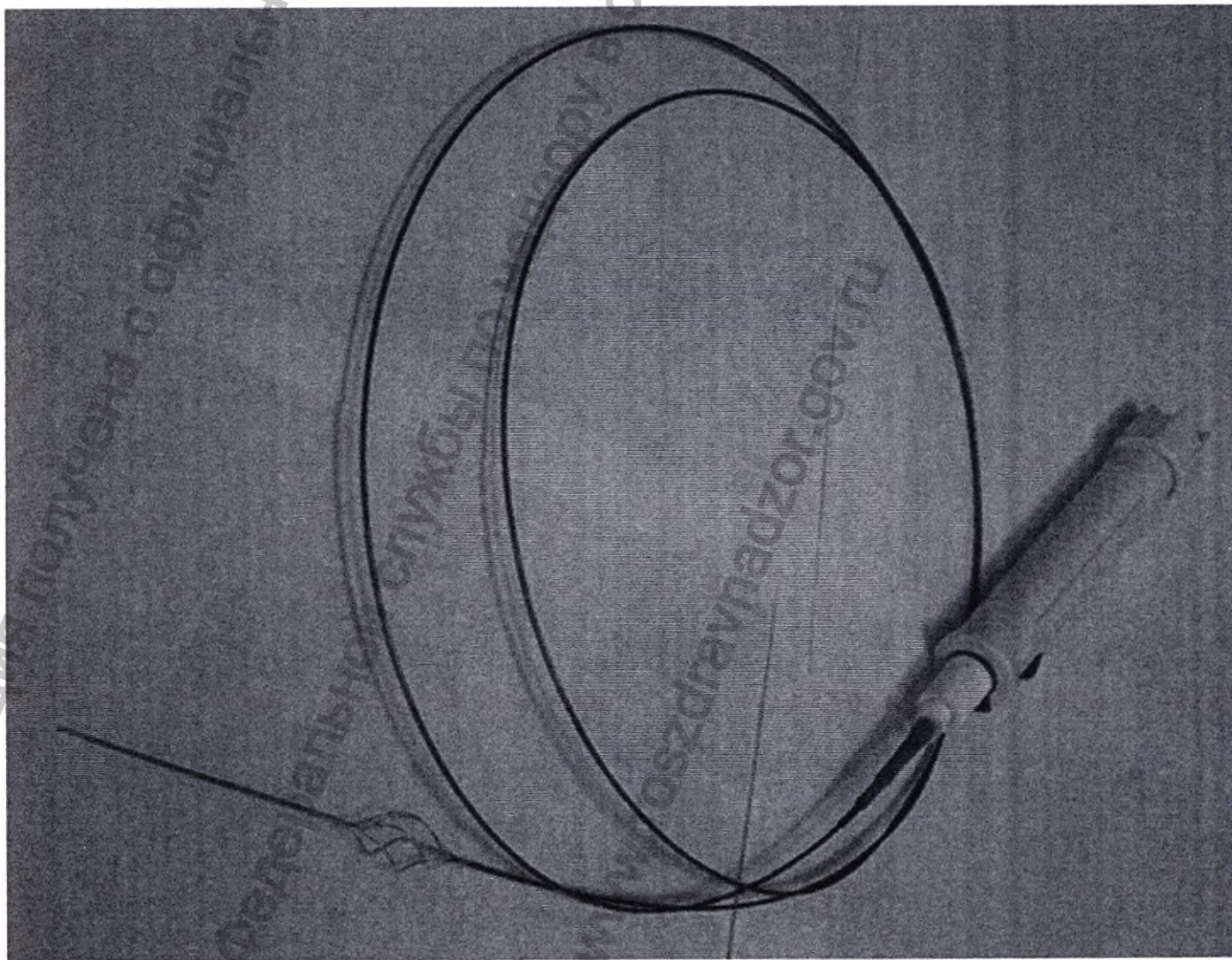
Рис. 16 Захваты типа «корзинка» спиралевидные для удаления камней Gemini 5 проволоки (нитевидный наконечник 5 см) 3F
