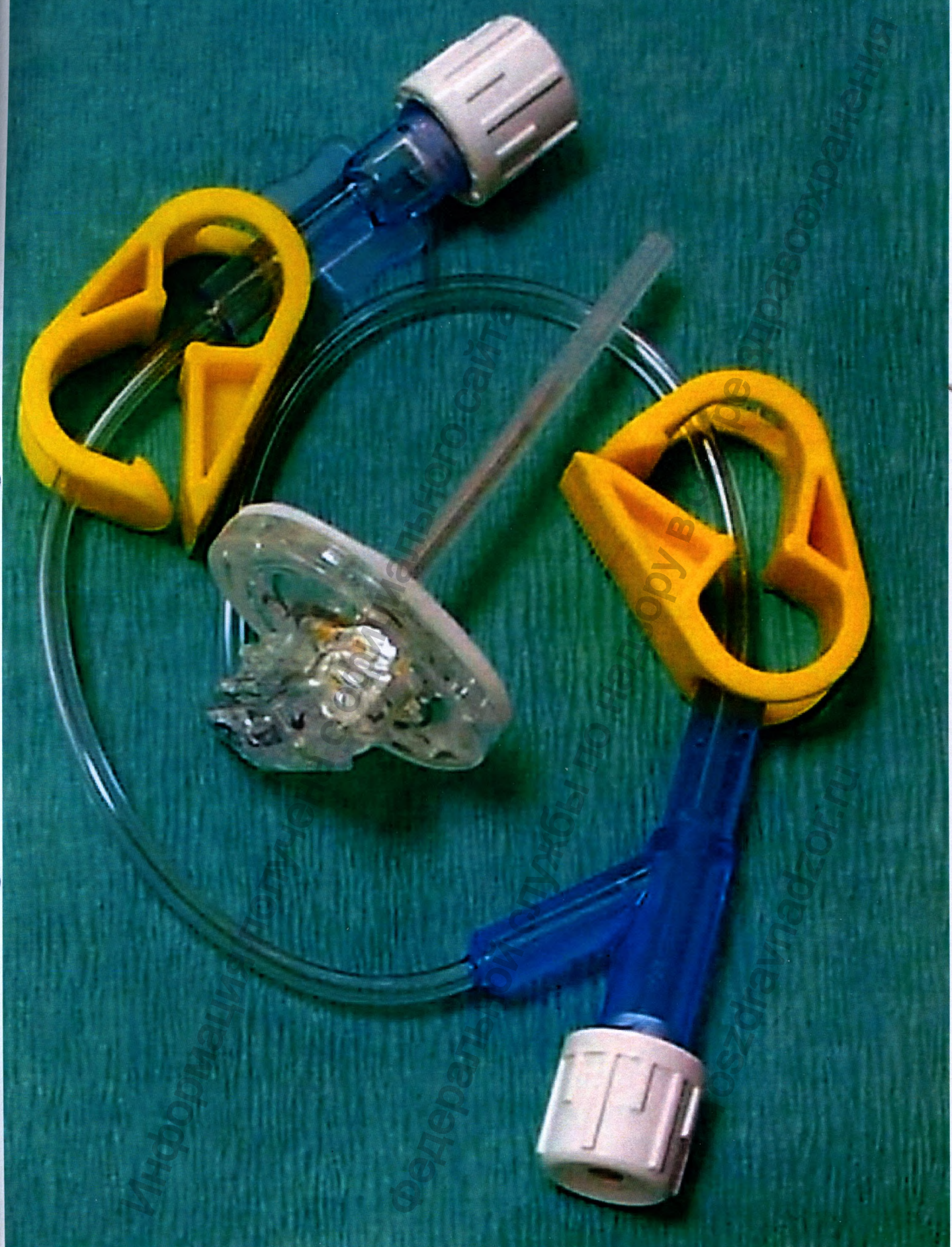
Игла Губера с предохранительным устройством и трубкой с Y-образным узлом или без него, размер иглы (один из): 0,9 мм x 19 мм, 0,9 мм x 25 мм, 0,9 мм x 38 мм из «Комплект инфузионный для автоматических инъекций PowerLoc Max»
