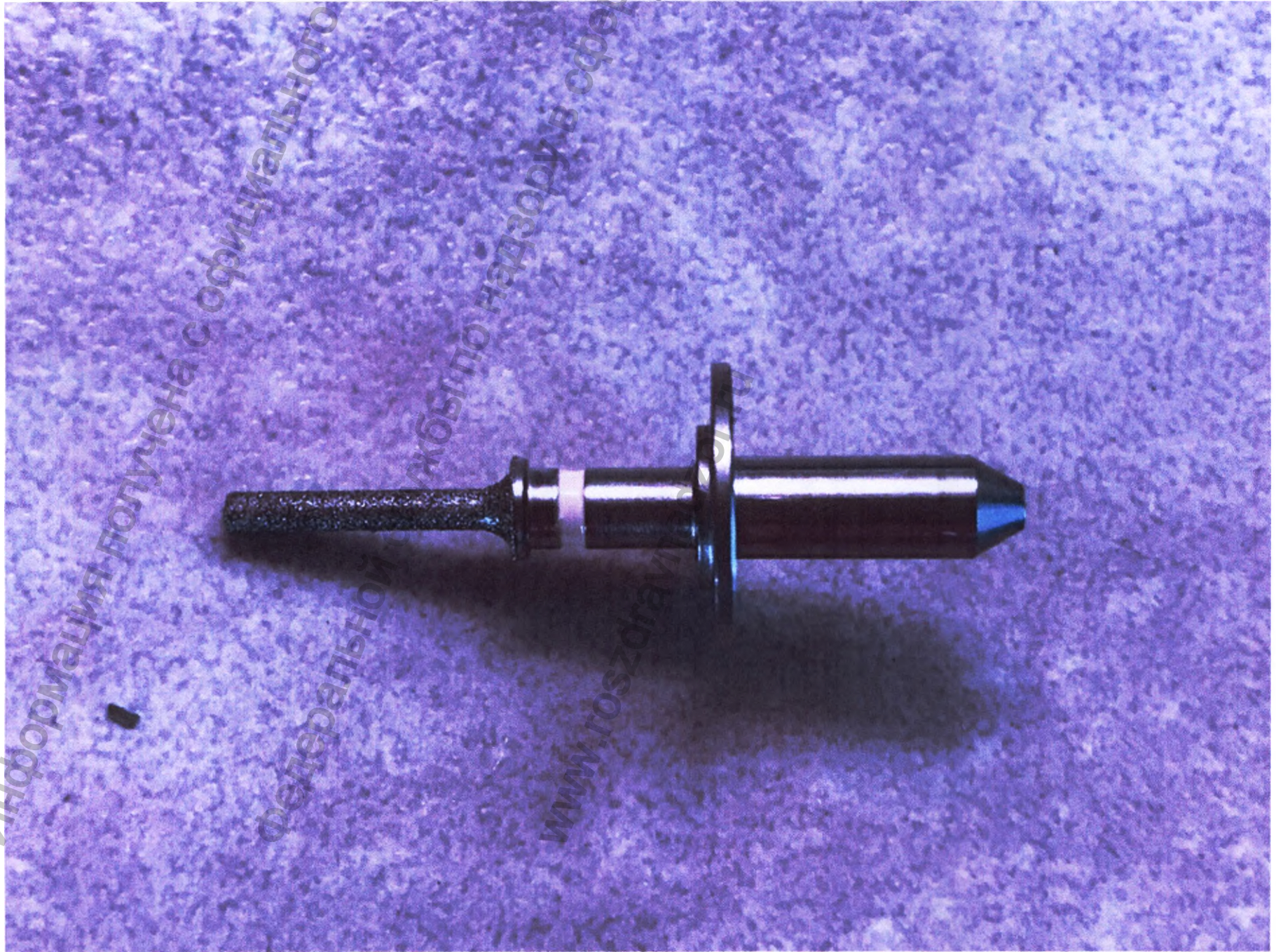
6.2. Фреза эллипсоидная (Ellipsoidal, 1 желтая полоска).
