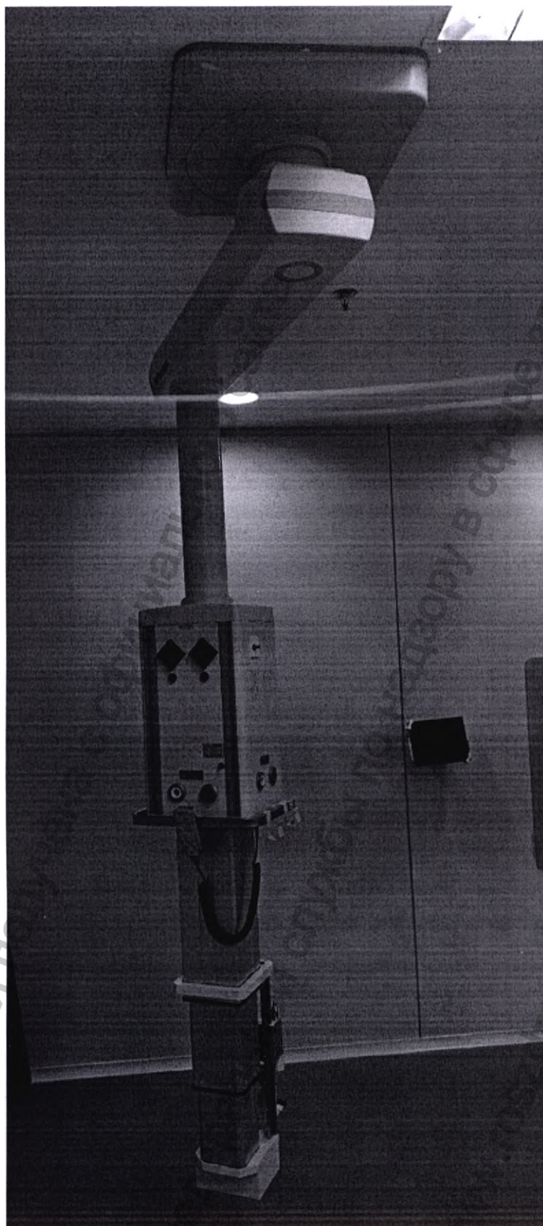
Консоль медицинская NuPort для подвода медицинских газов и подключения аппаратуры, с принадлежностями, вариант исполнения: NuPort 9000
