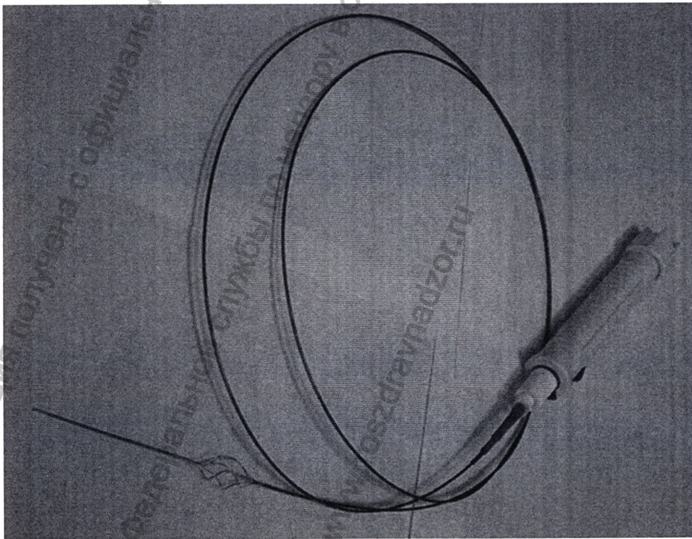
Рис. 16 Захваты типа «корзинка» спиралевидные для удаления камней Gemini 5 проволоч (нитевидный наконечник 5 см) 3F
