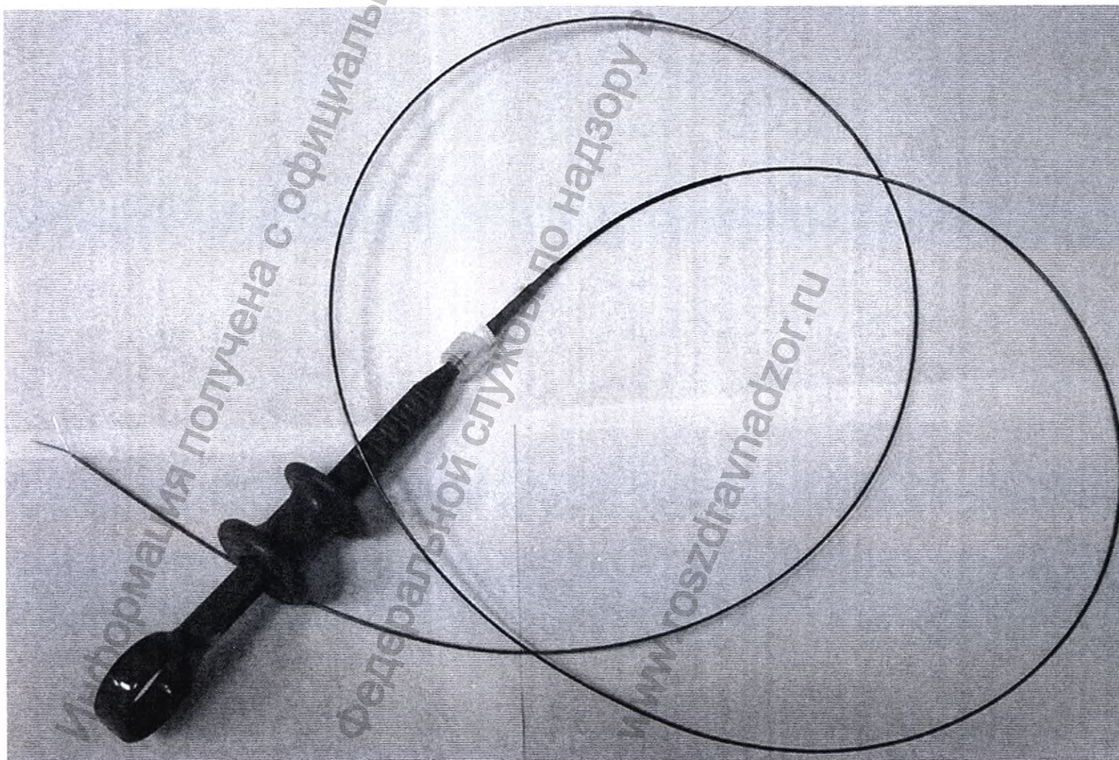
Рис. 2 Захваты крючкообразные для удаления камней Tricser (не ретрактирующие) 3F
