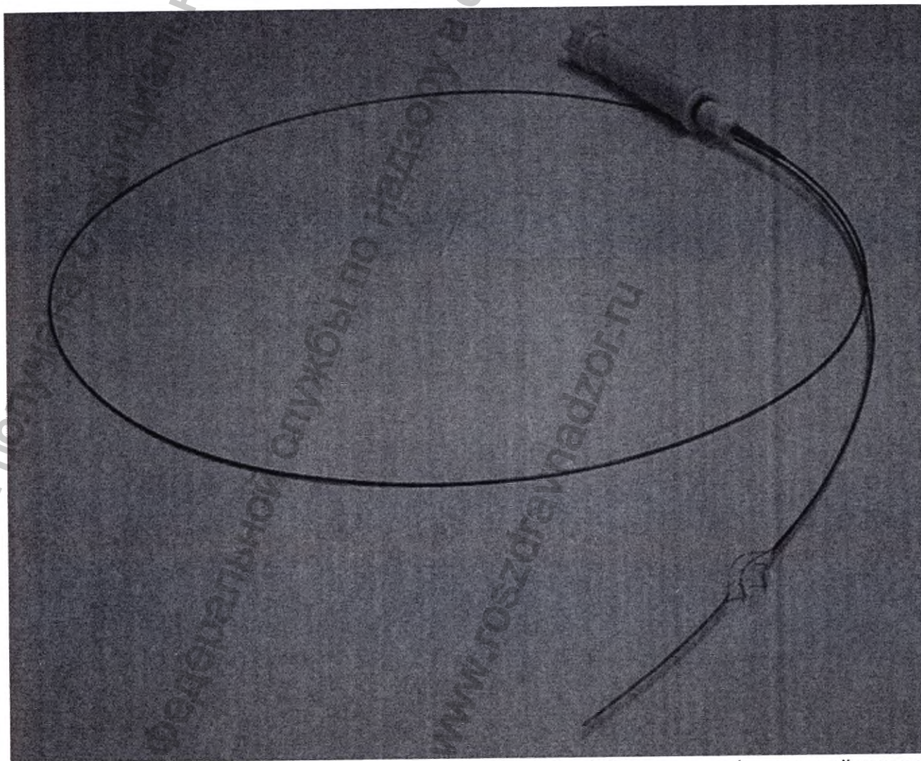
Рис. 14 Захваты типа «корзинка» спиралевидные для удаления камней Gemini 4 проволоки (нитевидный наконечник 5 см) ЗФ
