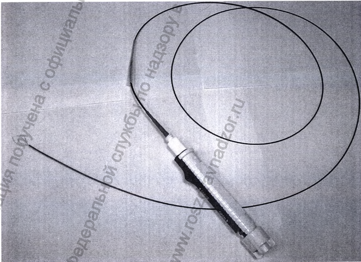
Рис. 5 Захваты нитиноловые для удаления камней Grasplit
