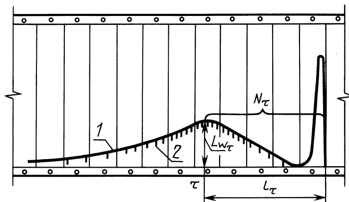
1 — кривая отклонения пера самописца; 2 — сброс пера самописца
