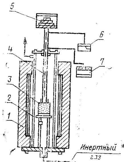
1—нагревательная печь; 2—нагревательная камера; 3—тигель с пробой; 4—шток с подпятником; 5—груз; 6—устройство регулировки и контроля температуры нагрева пробы; 7—прибор для автоматической записи температуры пробы и перемещения штока
